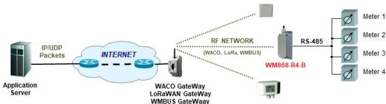
Obr. 1: Princip přenosu dat z modulu WM868-R4-B přes komunikační bránu
