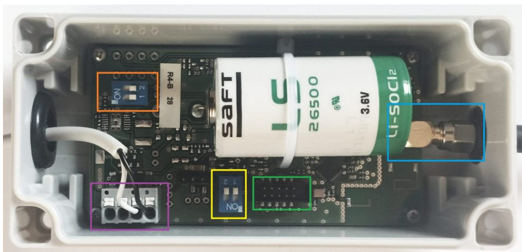
Obr. 10: Detailní pohled na modul WM868-R4-B
