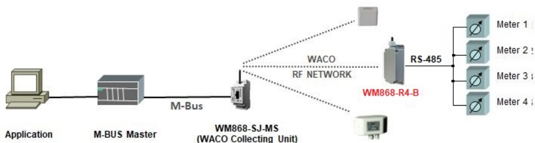
Obr. 2: Princip přenosu dat z modulu WM868-R4-B na jiný radiový modul WACO
