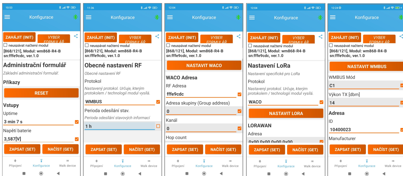
Obr. 4: Náhled formulářů pro nastavení komunikace modulu WM868-R4-B pomocí mobilní aplikace
