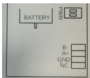
Obr. 12: Schéma zapojení připojovacích svorek modulu WM868-R4-B
