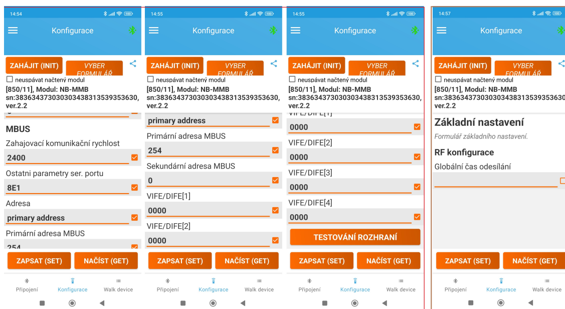
Obr. 4: Formuláře modulu NB-MM-V v aplikaci „SOFTLINK Konfigurátor” (3)
