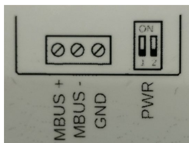
Obr. 9: Schéma připojení vodičů sběrnice M-Bus ke svorkovnici modulu NB-MM-V
