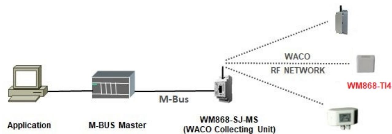
Obr. 2: Princip přenosu dat z modulu WM868-TI4 na jiný radiový modul WACO
