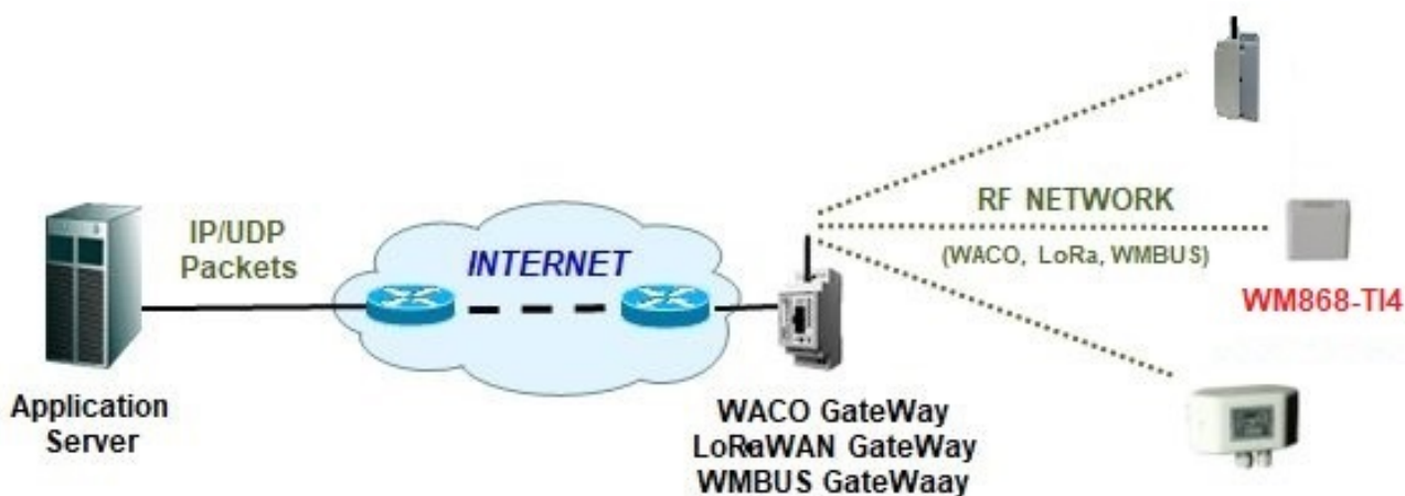
Obr. 1: Princip přenosu dat z modulu WM868-TI4 přes komunikační bránu
