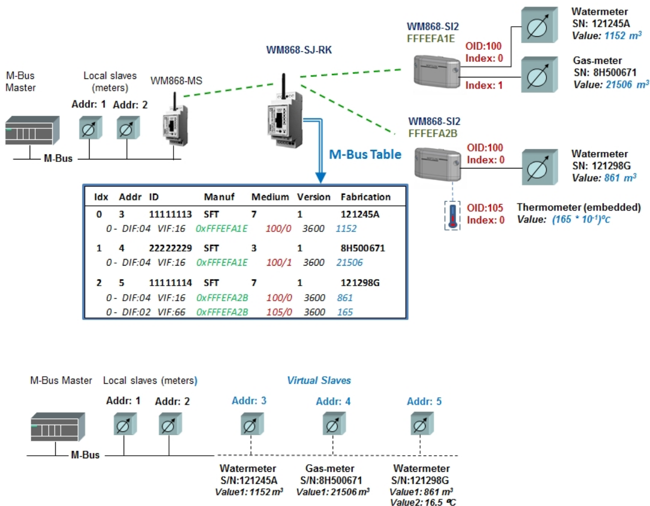
Obr. 19: Princip konverze dat sběrné jednotky WACO
