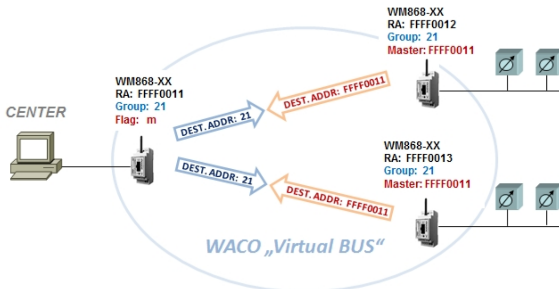
Obr. 16: Princip adresace v aplikaci „Virtual BUS” systému WACO
