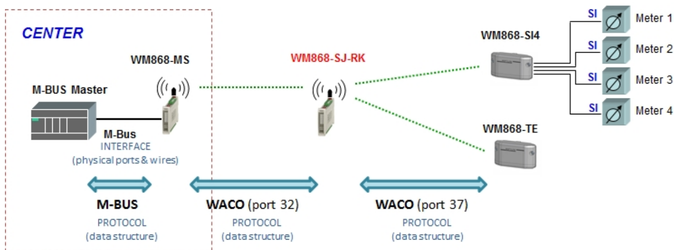
Obr. 1: Princip konverze dat sběrné jednotky WM868-SJ-RK
