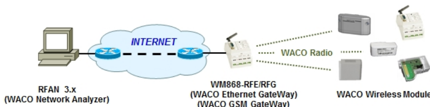
Obr. 8: Princip vzdálené konfigurace modulu
