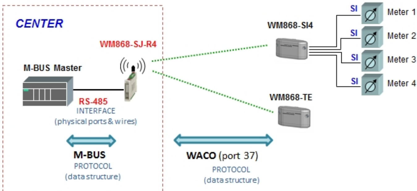
Obr. 1: Princip konverze dat sběrné jednotky WM868-SJ-R4
