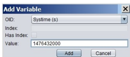
Obr. 16: Nastavení systémového času radiovou cestou
