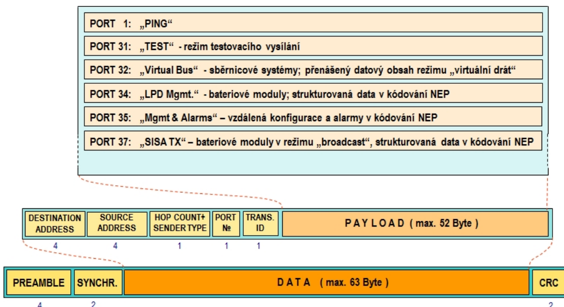
Obr. 19: Struktura datové zprávy systému WACO
