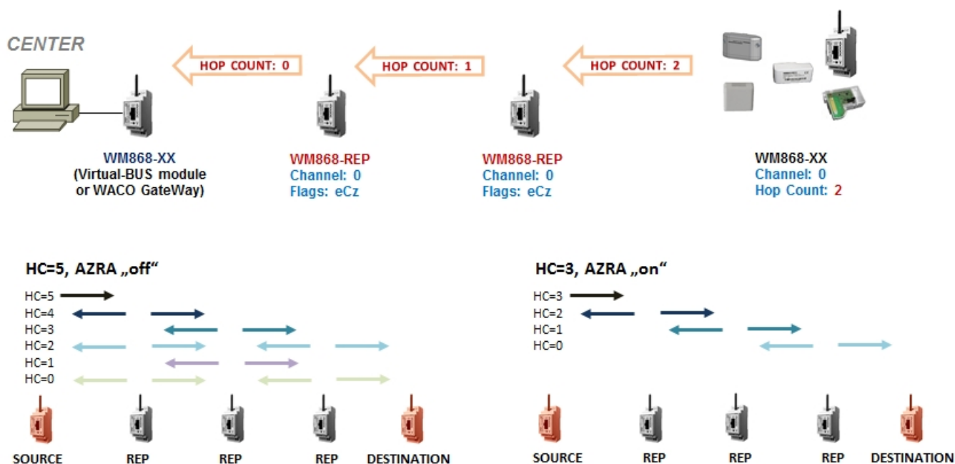
Obr. 1: Princip opakování zpráv v sítích WACO
