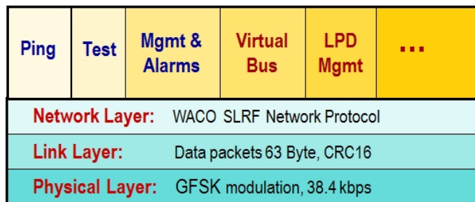
Obr. 18: Struktura komunikačních vrstev protokolu WACO SLRF
