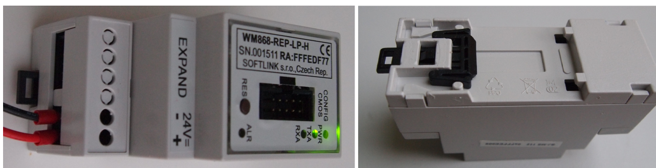
Obr. 20: Detailní pohled na modul WM868-REP-LP-H
