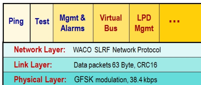
Obr. 19: Struktura komunikačních vrstev protokolu WACO SLRF
