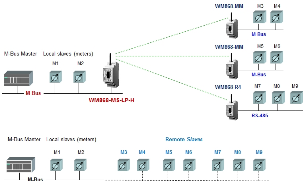
Obr. 1: Princip transparentního přenosu dat v síti WACO
