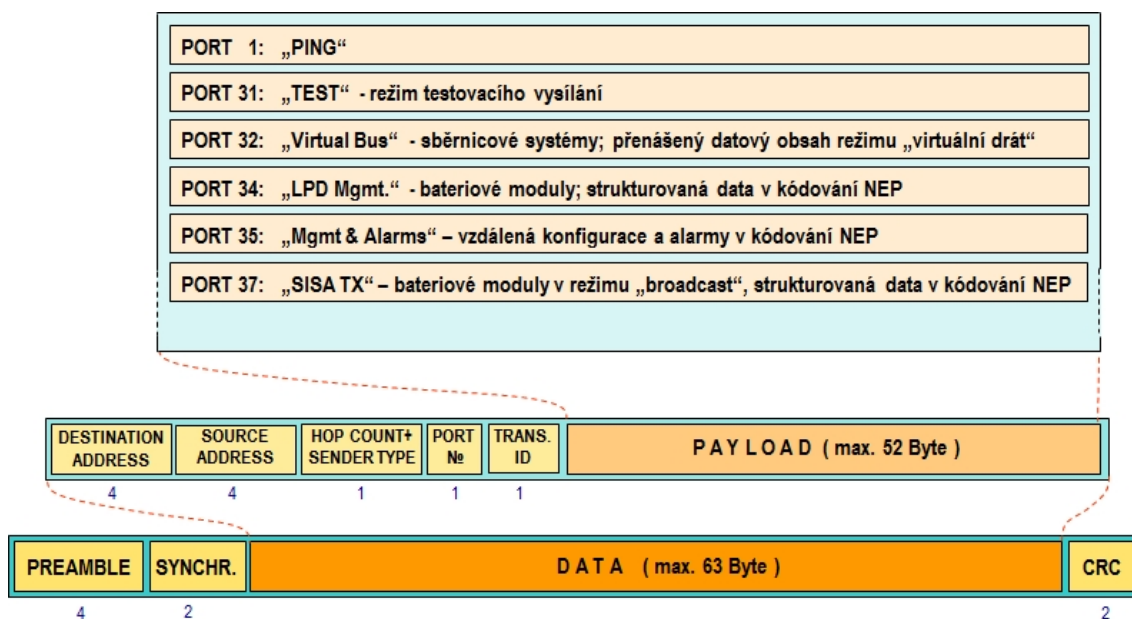
Obr. 20: Struktura datové zprávy systému WACO
