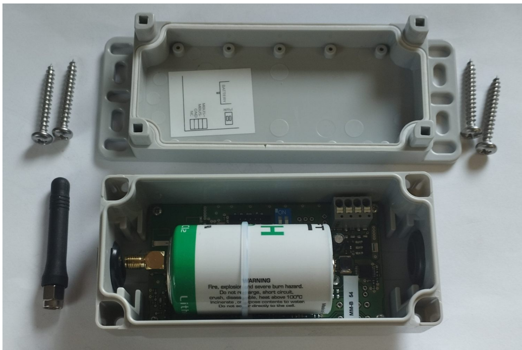
Obr. 11: Sestava modulu WM868-MM-B s tyčkovou anténkou
