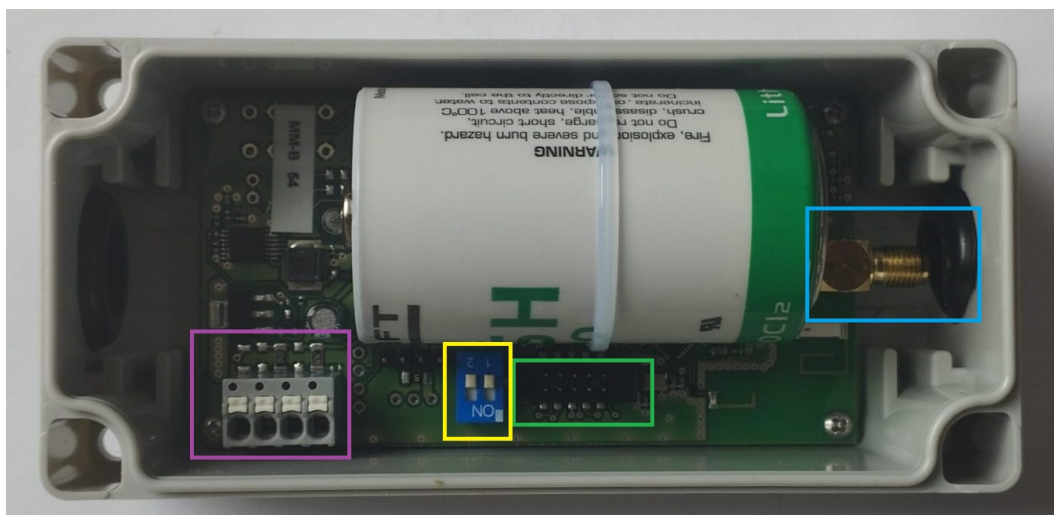
Obr. 10: Detailní pohled na modul WM868-MM-B
