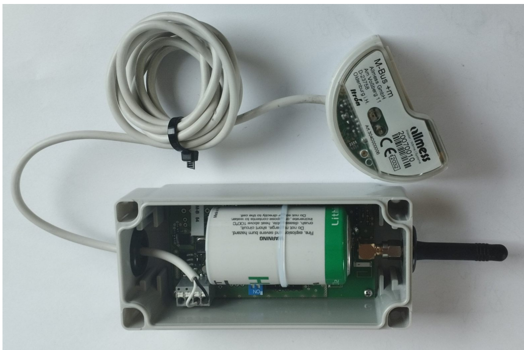
Obr. 13: Pohled na modul WM868-MM-B s připojenou anténou a zařízením M-Bus
