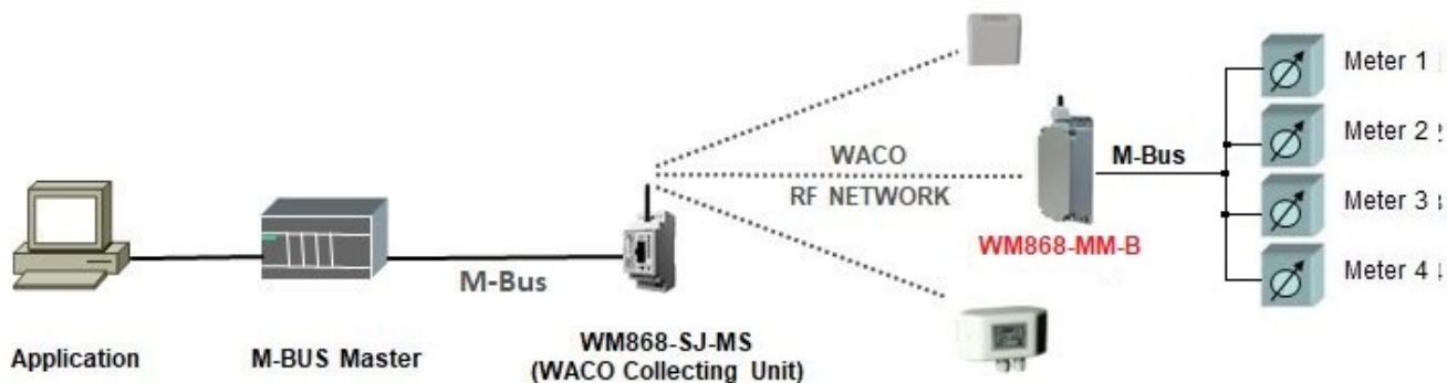
Obr. 2: Princip přenosu dat z modulu WM868-MM-B na jiný radiový modul WACO
