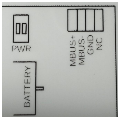
Obr. 12: Schéma zapojení připojovacích svorek modulu WM868-MM-B
