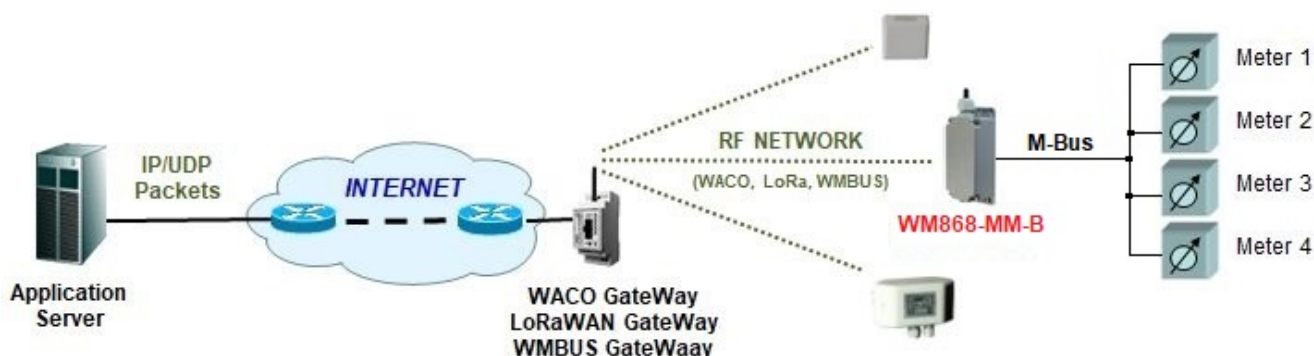
Obr. 1: Princip přenosu dat z modulu WM868-MM-B přes komunikační bránu
