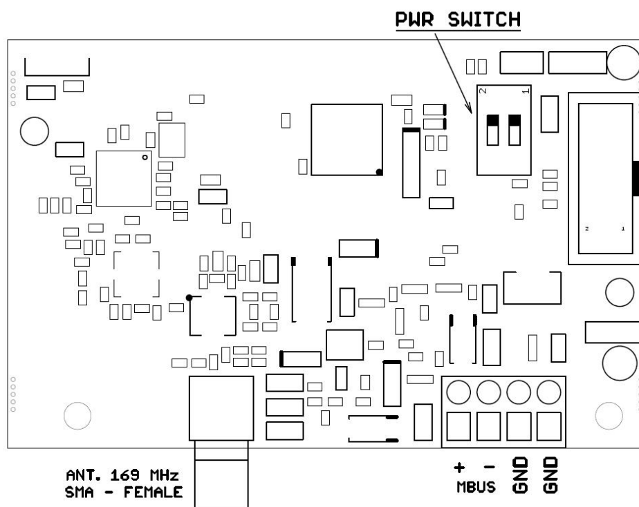
Obr. 9: Rozmístění elementů desky plošného spoje modulu WB169-MMB
